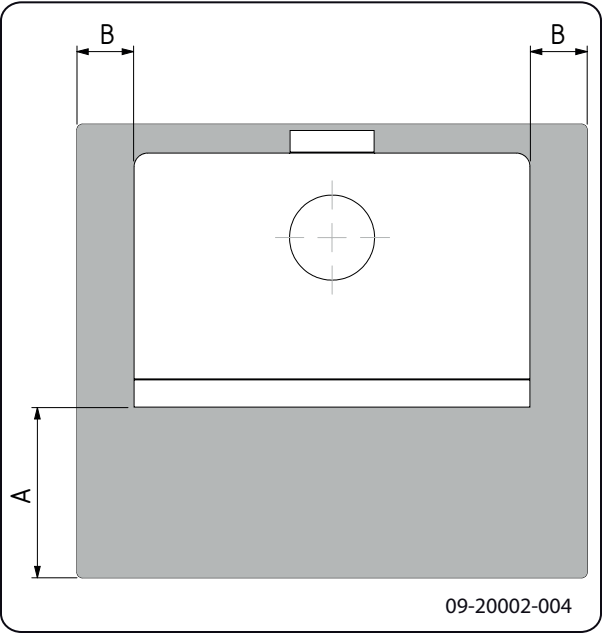
Dimensiones mínimas de la placa de apoyo ignífuga
